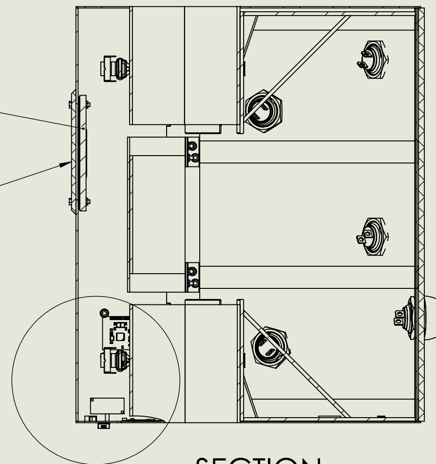
SECTION D-D SCALE 1 : 5
